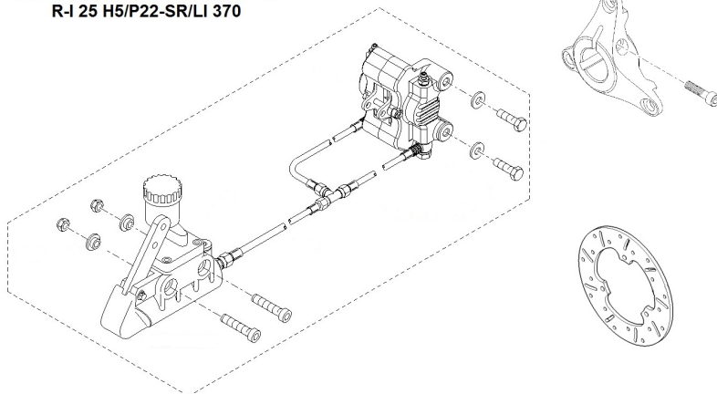
IMPIANTO FRENO EASYKART 60 R-I 25 H5/P22-SR/LI 370
