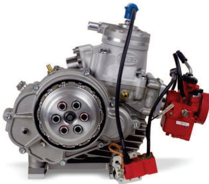
FOTO MOTORE LATO FRIZIONE PHOTO OF OPPOSITE SIDE OF ENGINE
