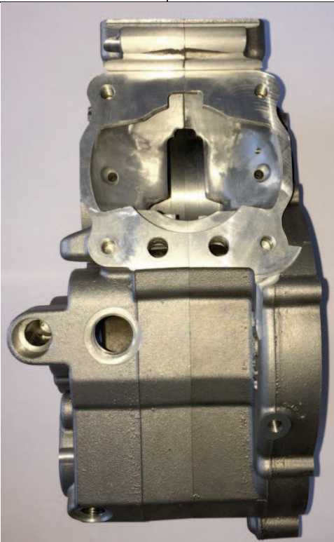
FOTO CARTER (GUARNIZIONE BASE)
